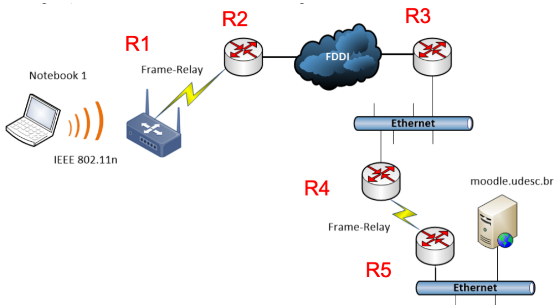
Figura 1 – Topologia da Rede
